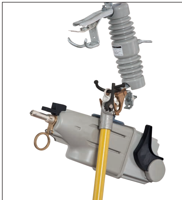
Figura 13. Elevar el TripSaver II fuera del montaje utilizando una pértiga de gancho.
