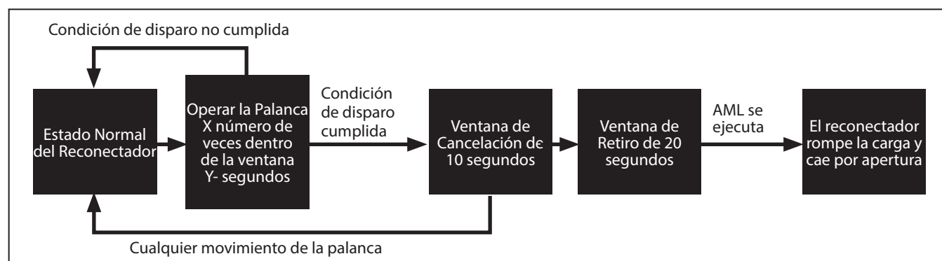
Figura 35. Como trabaja la función AML.
