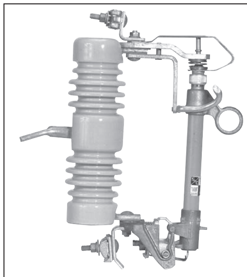
Figura 2. Producción anterior (“-R9”) montaje en cortacircuito de S&C. “-R8” y versiones anteriores tienen un contacto superior similar.
