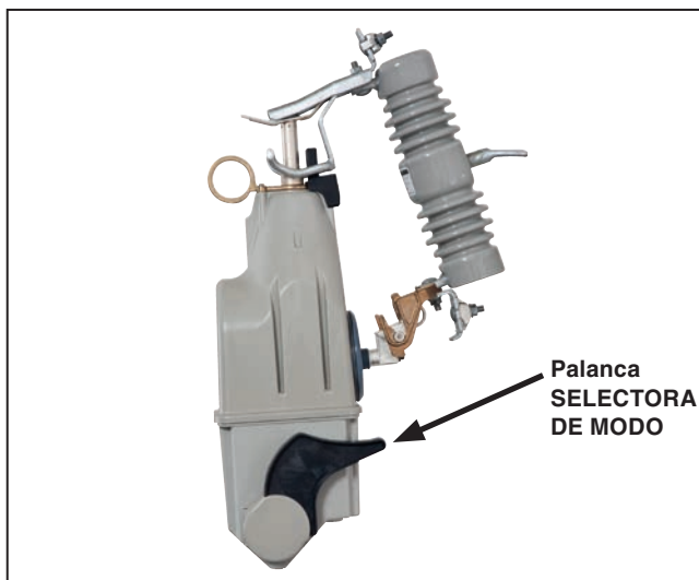
Figura 7. Palanca SELECTORA DE MODO en la posición Auto.
