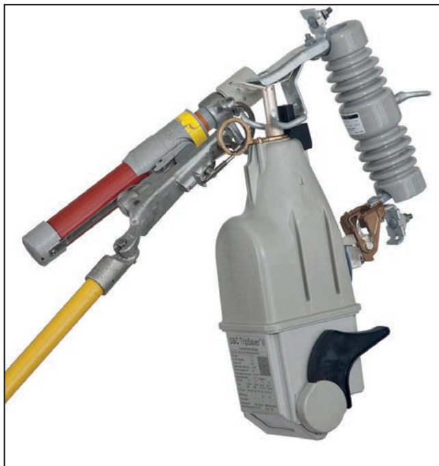
Figura 31. La herramienta Loadbuster sujeta a un Reconectador Montado en Cortacircuito TripSaver II.
