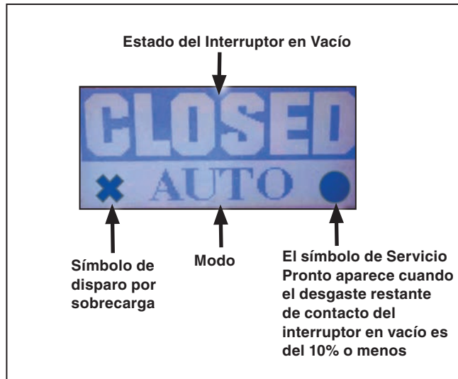
Figura 18. Ilustración de la pantalla Normal Primaria .
