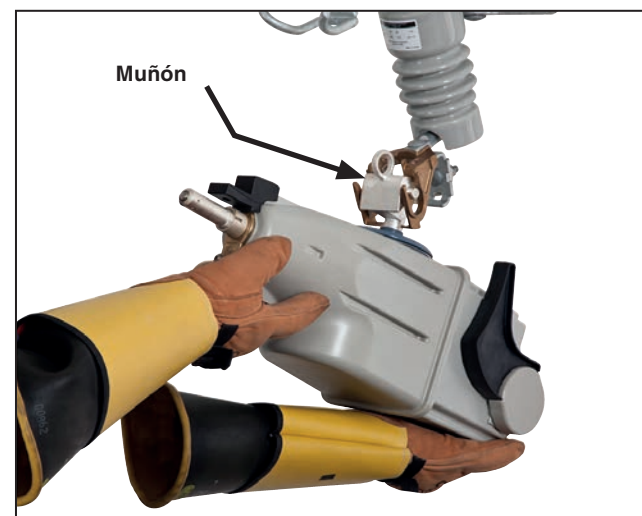
Figura 4c. Guiando el muñón dentro de la bisagra del montaje en cortacircuito.
