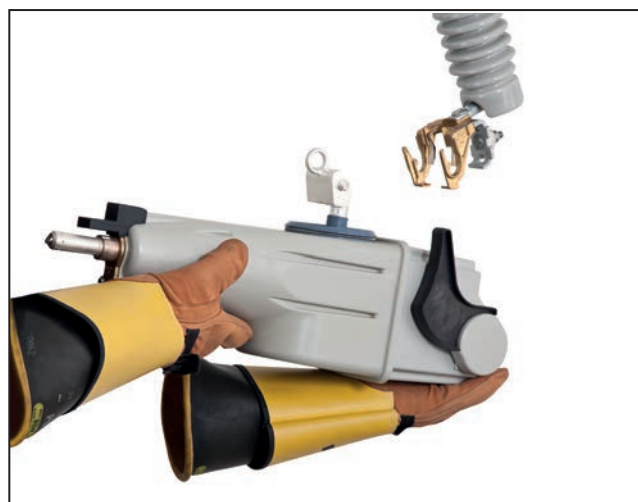
Figura 5b. Insertando un TripSaver II de 25 kV dentro de su montaje con las manos enguantadas.
