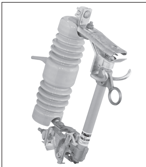
Figura 1. Producción actual (“-R10” o “-R11”) proporcionada por S&C de montaje en cortacircuito.
