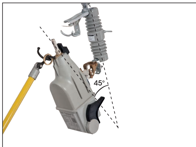
Figura 6. Oscile la unidad TripSaver II hasta más o menos 45 grados de la posición de Cerrado total antes del cierre final.
