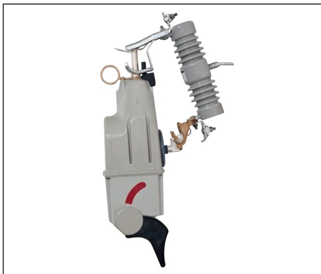
Figura 8. Palanca SELECTORA DE MODO en la posición NR.
