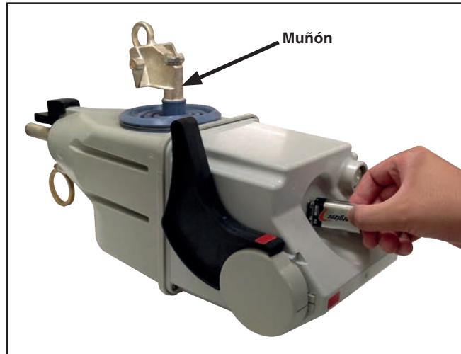
Figura 43. Reajustando manualmente el Reconector Montado en Cortacircuito TripSaver II.
