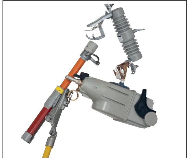
Figura 33. Desprendiendo una herramienta Loadbuster de un reconectador TripSaver II.
