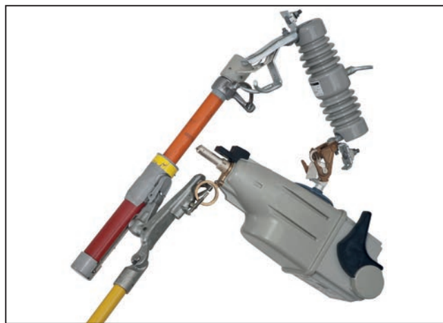
Figura 32. Una herramienta Loadbuster en la posición de Disparo.
