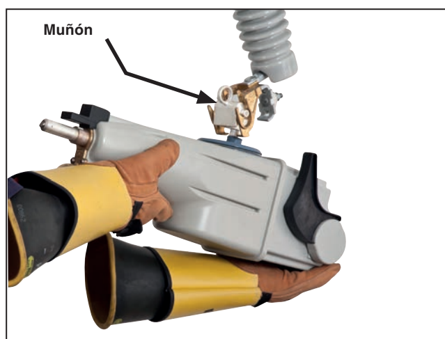
Figura 5c. Guiando el muñón dentro de la bisagra del montaje en cortacircuito.
