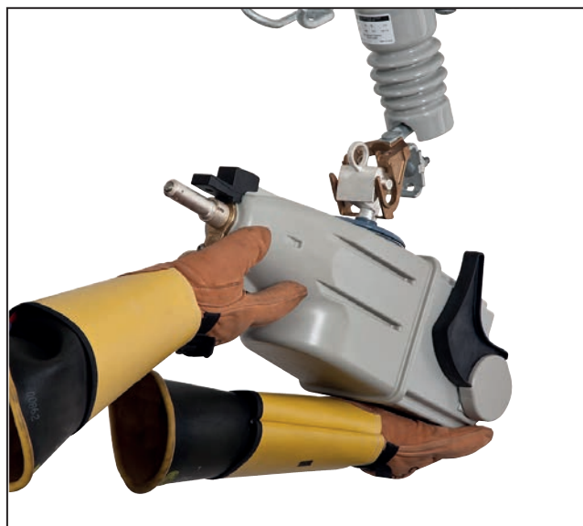
Figura 14. Elevar la unidad TripSaver II fuera del montaje utilizando las manos enguantadas.
