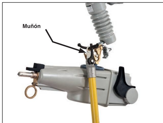
Figura 5a. Insertando un TripSaver II de 25 kV dentro de su montaje con una Herramienta de Manipulación Talon de S&C.
