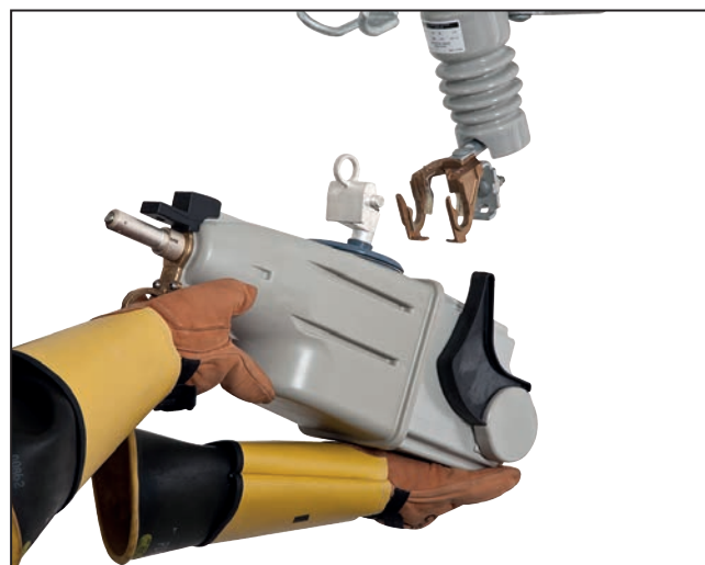
Figura 4b. Insertando el reconectador TripSaver II de 15 kV dentro de su montaje con las manos enguantadas.
