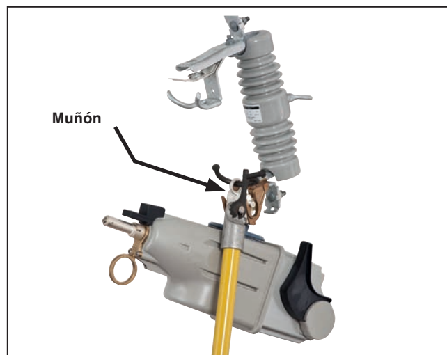
Figura 4a. Insertando el reconectador TripSaver II de 15 kV dentro de su montaje con una Herramienta de Manipulación Talon de S&C.
