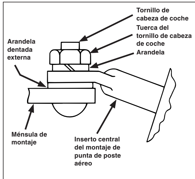
Figura 3. Sujeción de un montaje de TripSaver II Estilo Aéreo para Punta de Poste a la ménsula de montaje.
